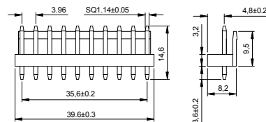
3962S-10P针座
